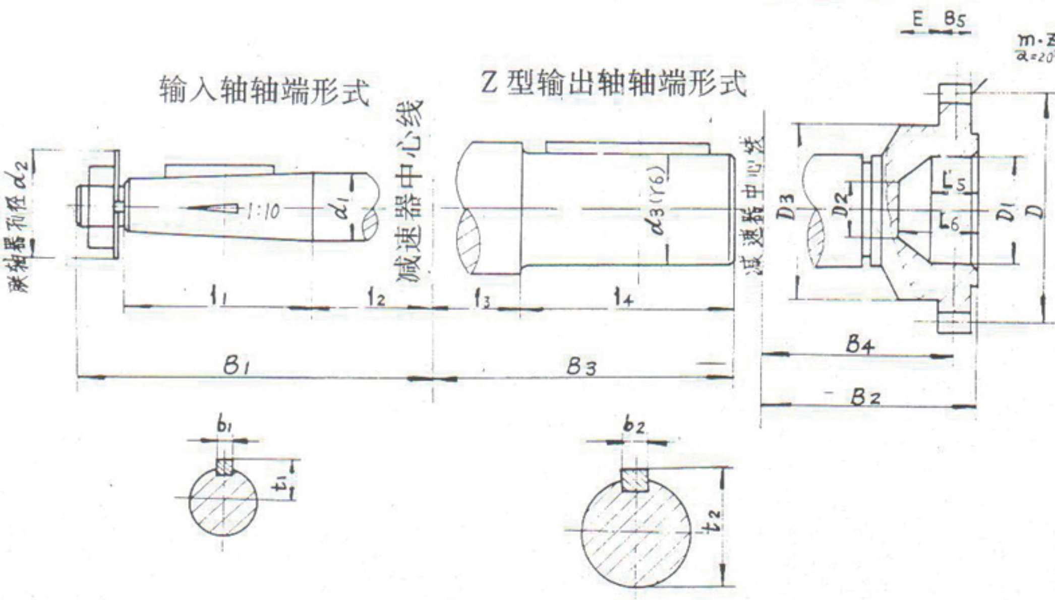
CA 型输出轴轴端形式
